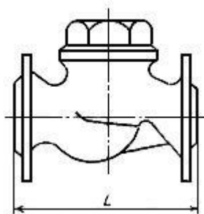
Клапан обратный проходной фланцевый с крышкой на резьбе
